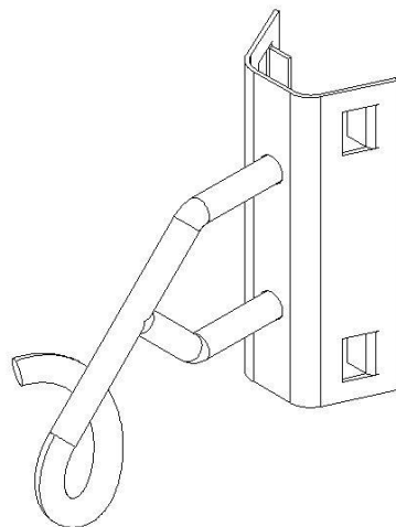
Эскиз изделия:
